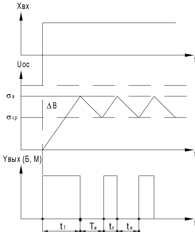
Рисунок 1.4 – Графики работы канала регулирования
